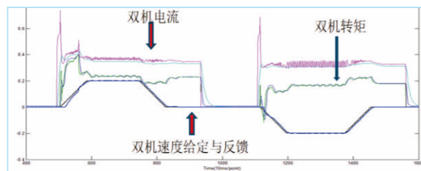
主从速度控制+从机转矩调节
