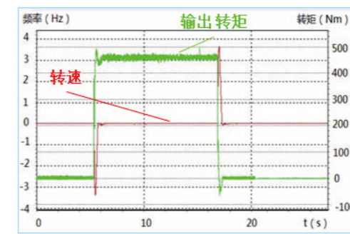
额定转矩230Nm，闭环0rpm时输出转矩为200% (45kW变频器控制37kW电机，电机额定转矩230Nm)
