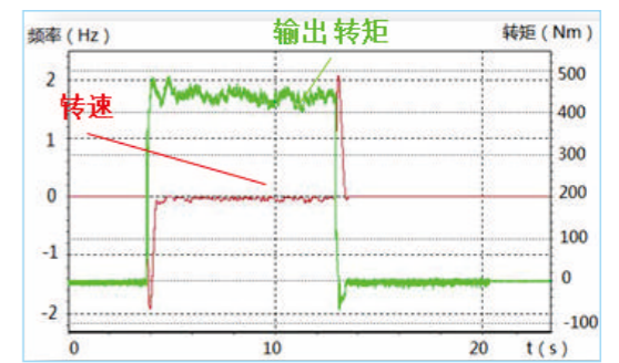
额定转矩230Nm，开环0rpm时输出转矩为200% (45kW变频器控制37kW电机，电机额定转矩230Nm)
