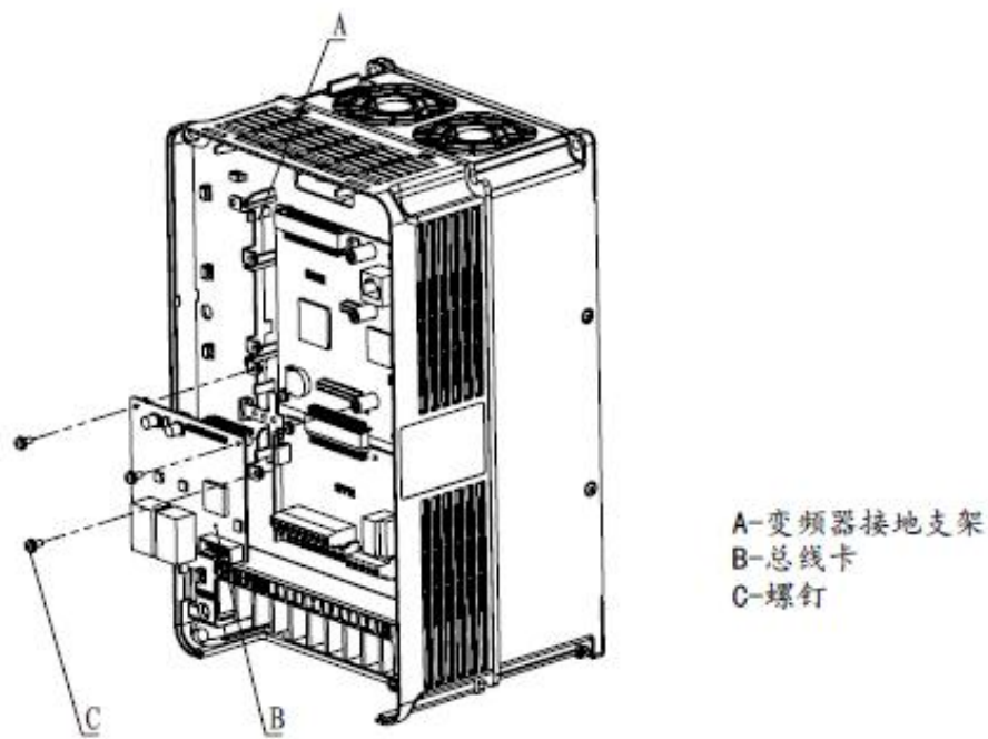
图 2 总线卡的安装与接地
