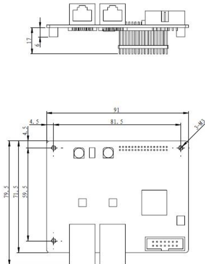
图 5 Modbus-Tcp 模块尺寸 (单位 mm)
