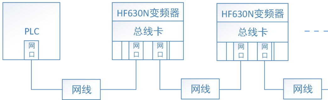
图 3 标准 Modbus-Tcp 电缆接线图
