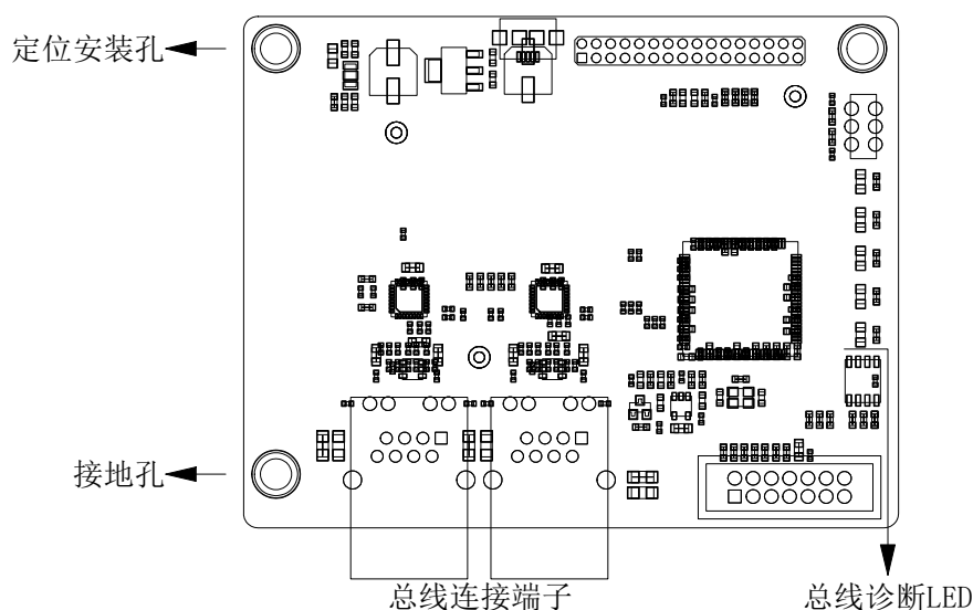
图 1 GDHF-AMTX2 总线卡布局图
