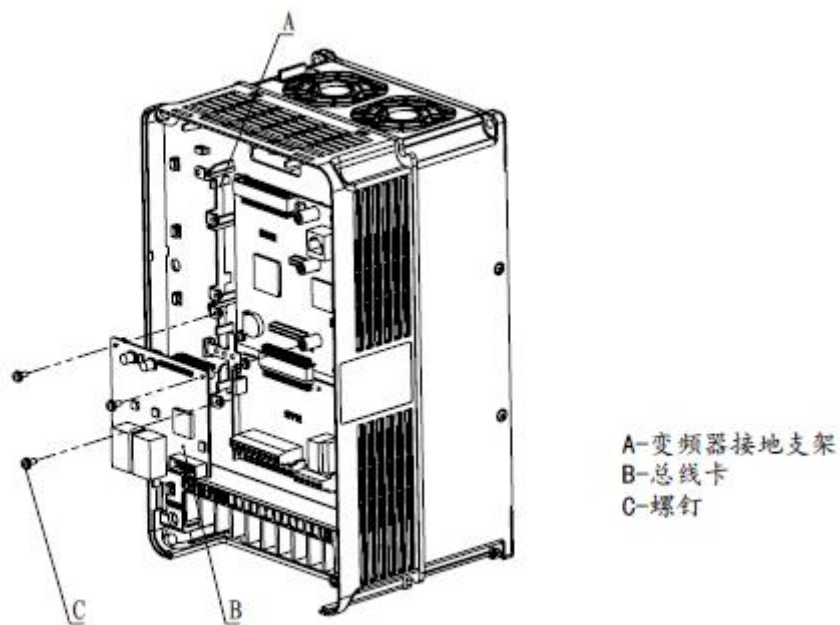
图 2 总线卡的安装与接地
