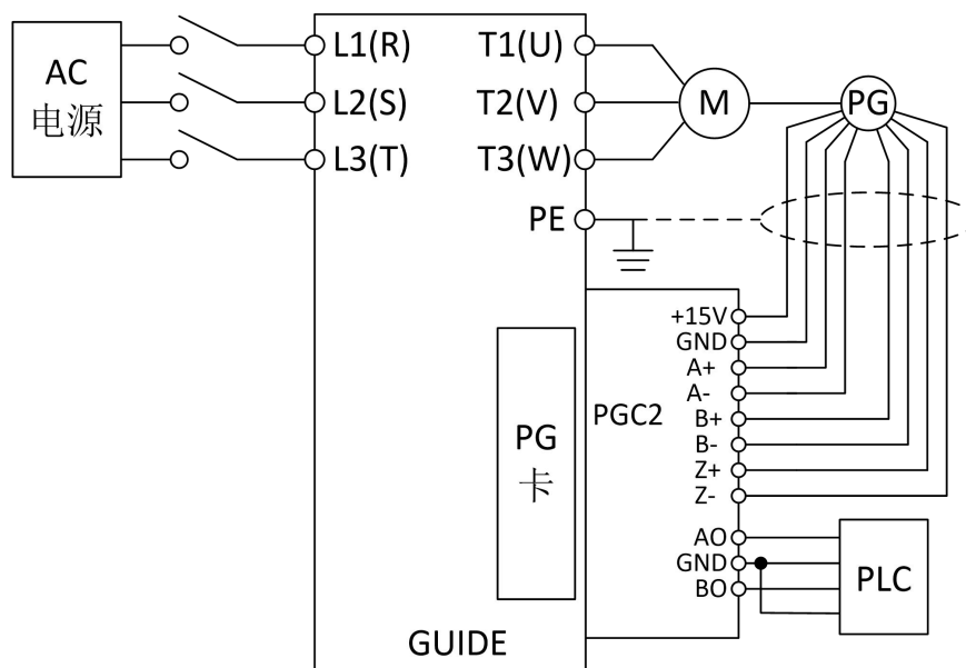
PGC2 卡接线原理示意图：
